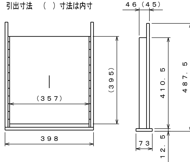
引出し (S=1:10)
