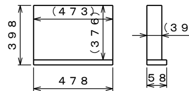
引出詳細図※ ( ) 寸法は内寸
