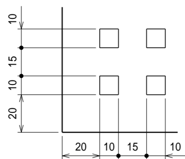
A部拡大図 S = 1 : 2
